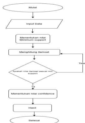
Gambar 2. Tahapan Algoritma Apriori
