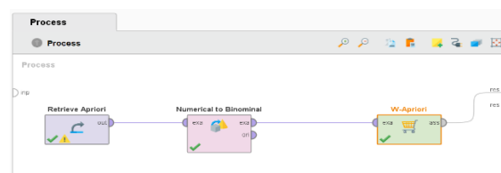
Gambar 3. Proses Algoritma Menggunakan W-Apriori
